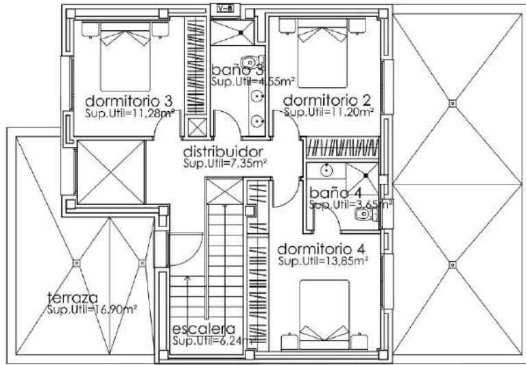
PLANTA PRIMERA
