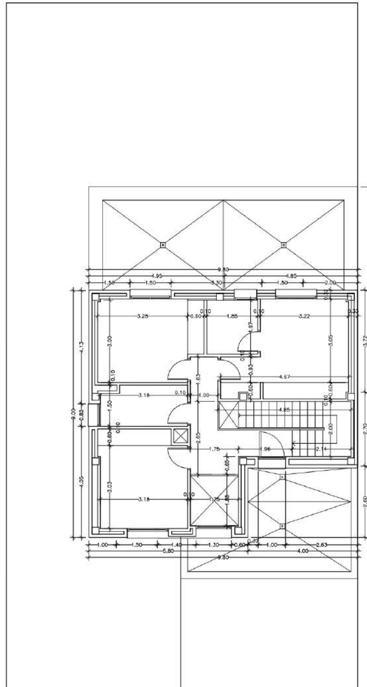
PLANTA PRIMERA. VIVIENDA TIPO
