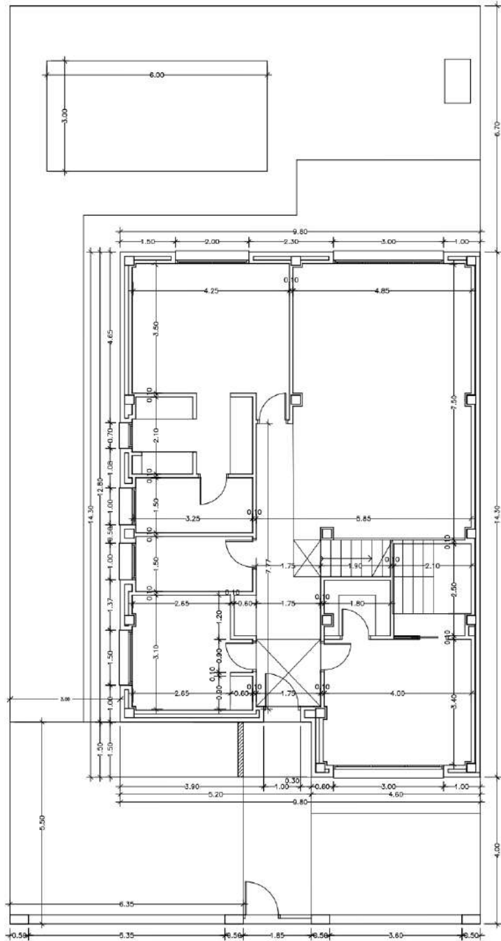
PLANTA BAJA. VIVIENDA TIPO
