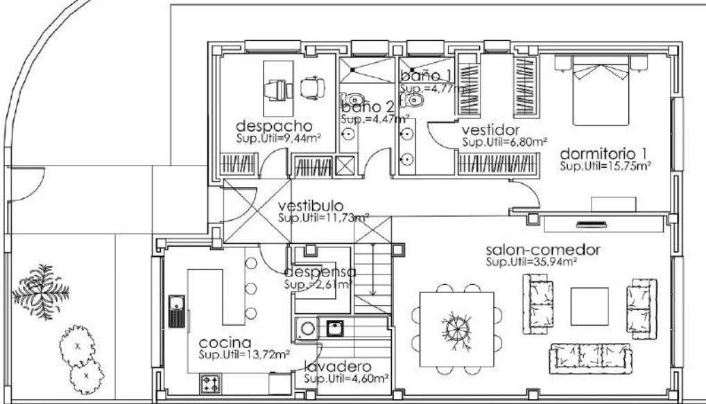
PLANTA BAJA
